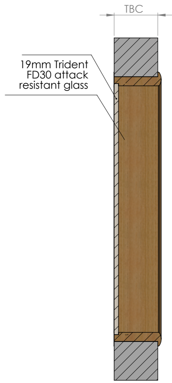
SECTION A-A
